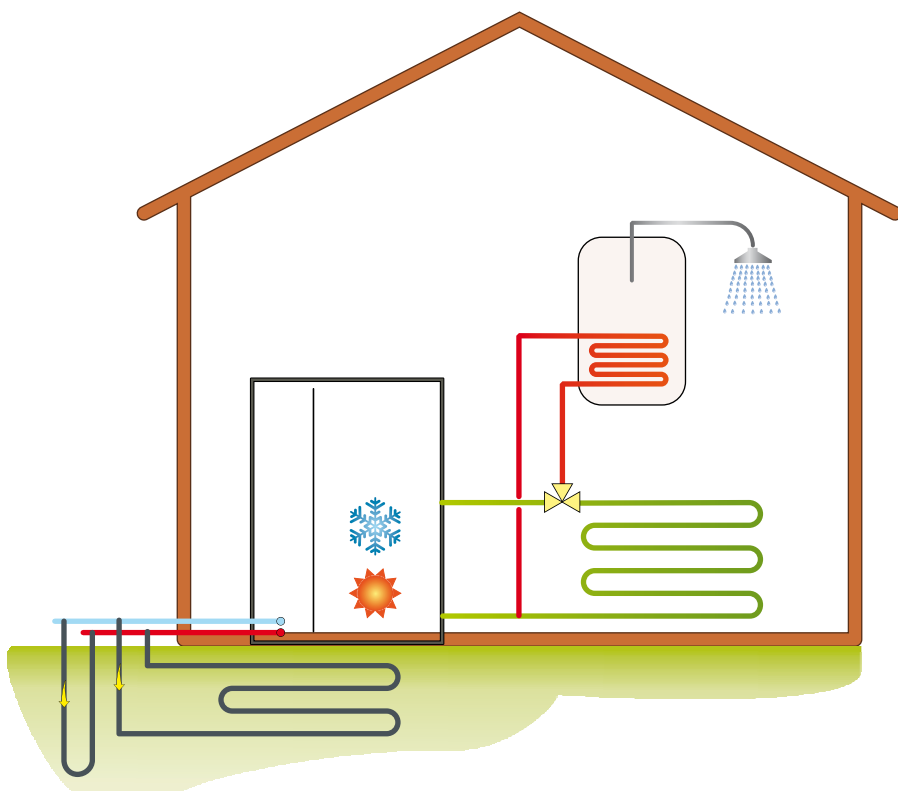
WZH/RV VERSIONE 2 TUBI. L'unità è in grado di produrre acqua refrigerata nel periodo estivo utilizzando l'inversione sul circuito frigorifero.
